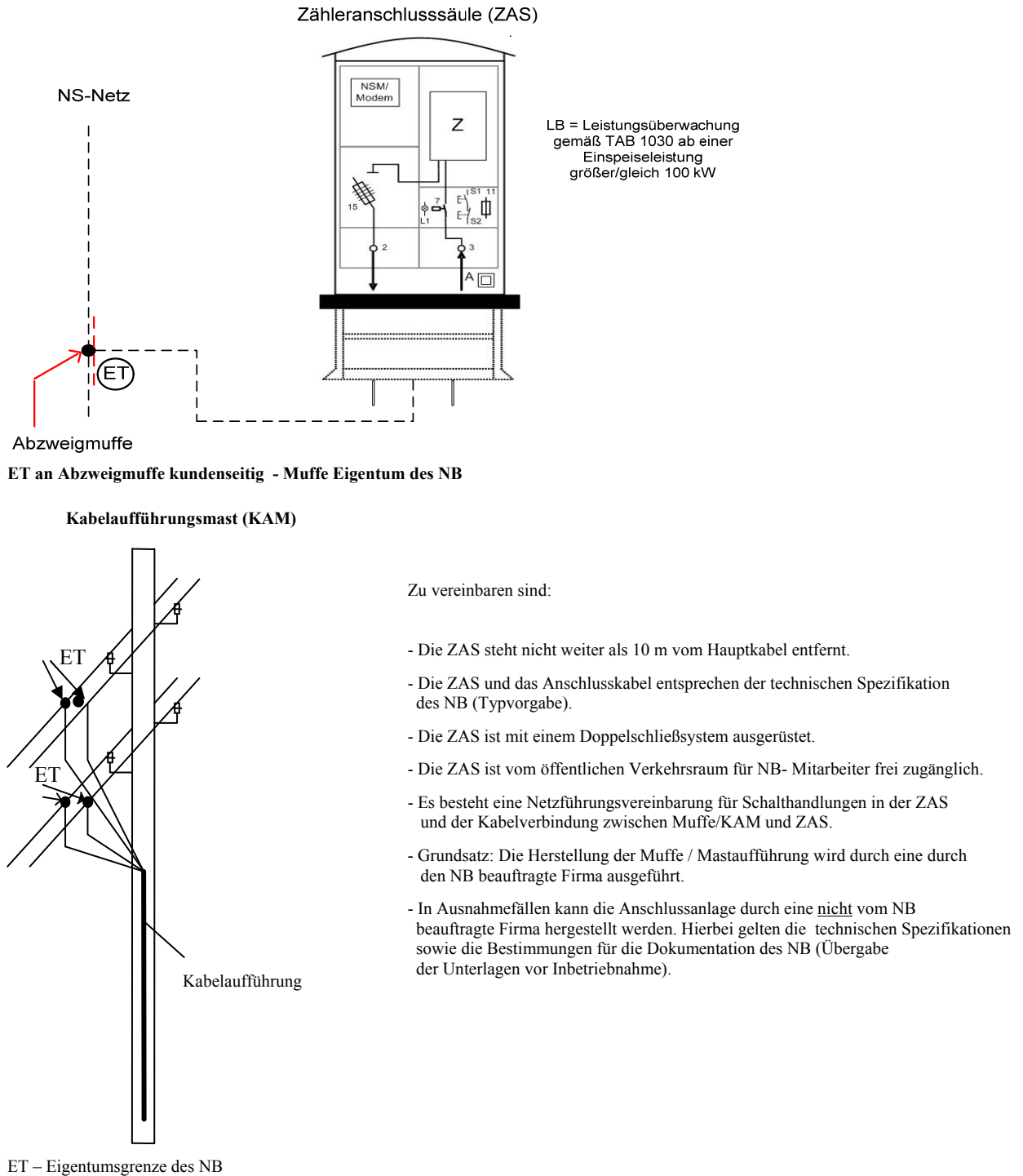
Bild 1 Erzeugungsanlage im Parallelbetrieb > 30KVA Anschluss mittels Abzweigmuffe oder Kabelaufführung bei Freileitung
