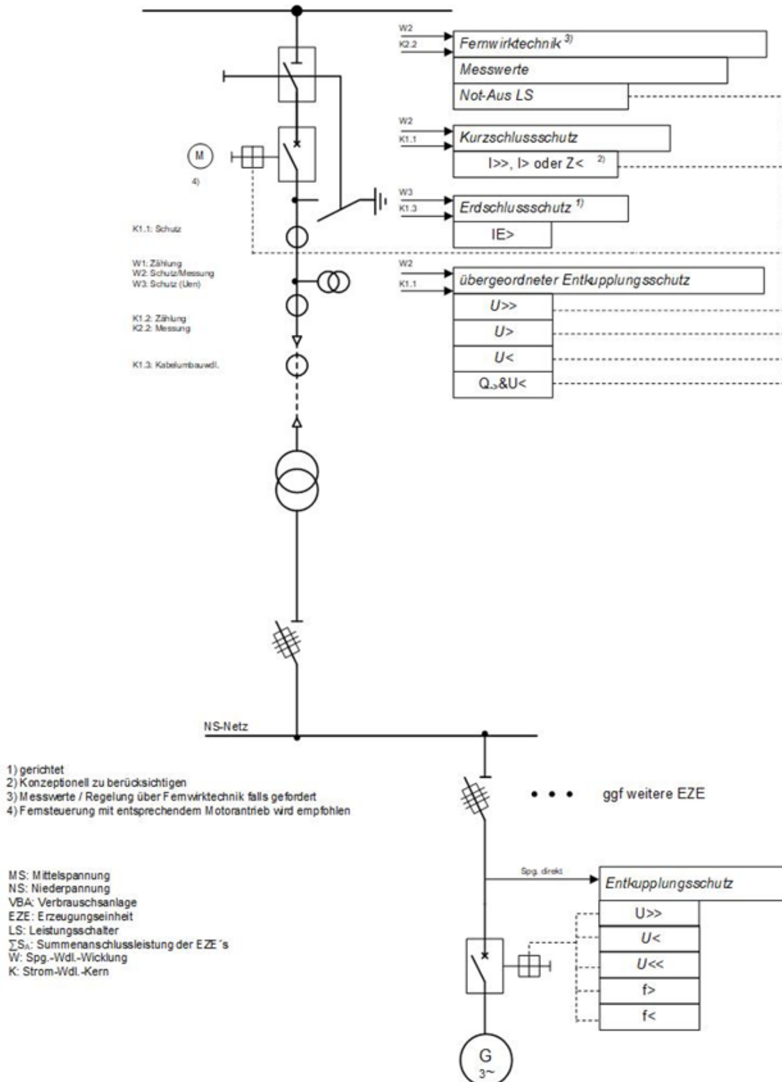
Bild 10 Einspeisung – Beispiel einer an das Mittelspannungsnetz angeschlossene Erzeugungsanlagen mit Leistungsschalter und Erzeugungseinheit ohne Inselbetriebsmöglichkeit
